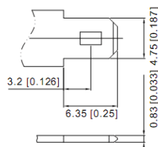
F1 (Faston Tab 187)
